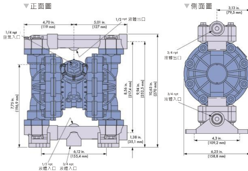
外型尺寸圖
